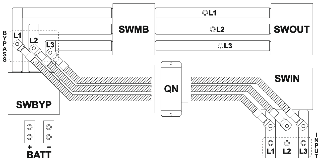
125KVA - BYPASS-ANSCHLUSS AN EINGANGSLEITUNG
