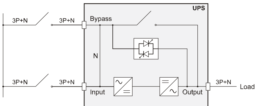
UPS sin variación de régimen de neutro y con ingreso bypass separado.
