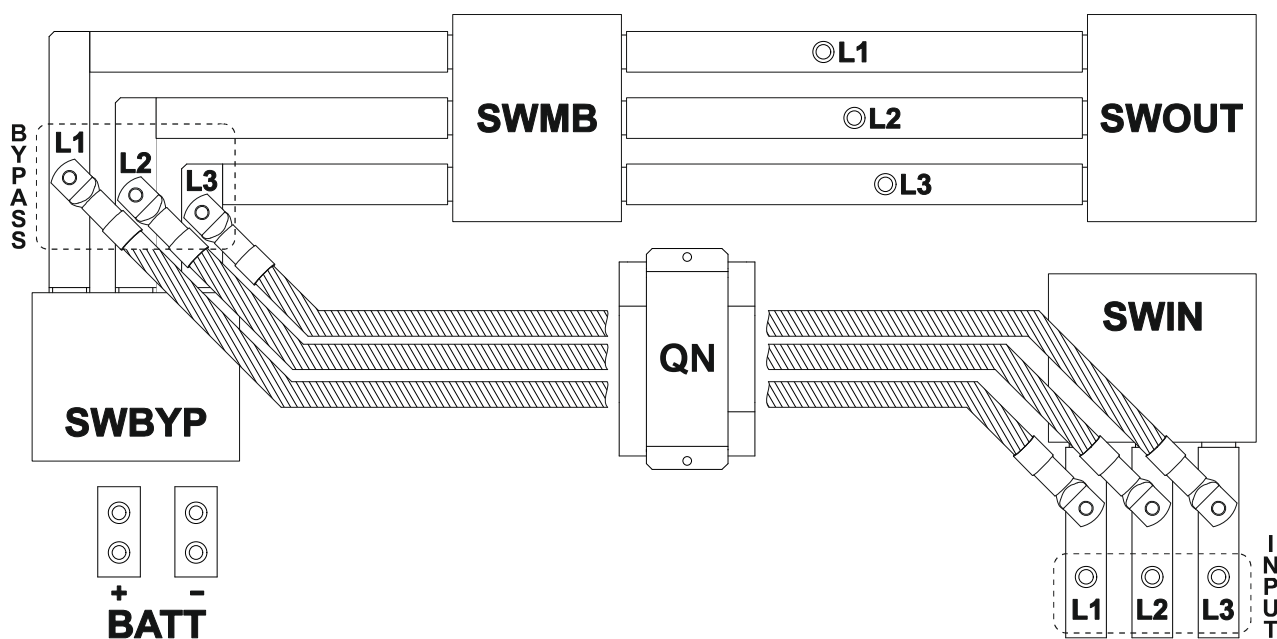
125KVA - BY-PASS CONNECTÉ À LA LIGNE D'ENTRÉE
